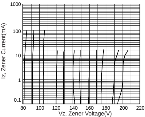
Fig. 4 - Vz=82 Thru 200 Volts
