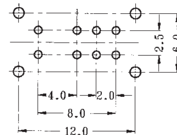
P.C.B. LAYOUT
