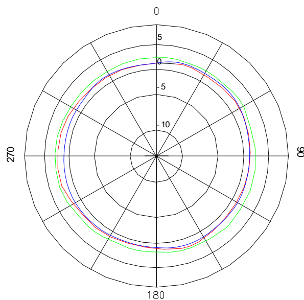
水平面方向图(2.4G天线) Horizontal Pattern
