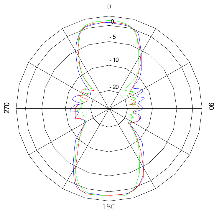
垂直面方向图 Vertical Pattern
