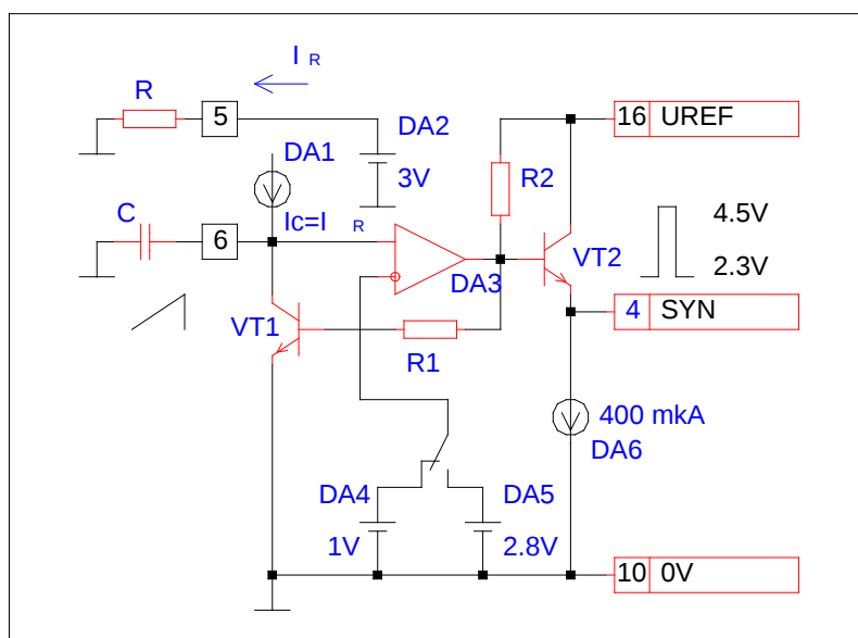
Рис. 5. Задающий генератор.
