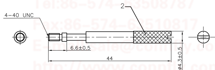
Long BOLT
