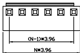
V/T Type
