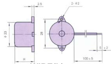
WIRE(L) type
