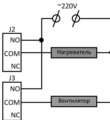
Рис. 3. Подключение нагрузки.
