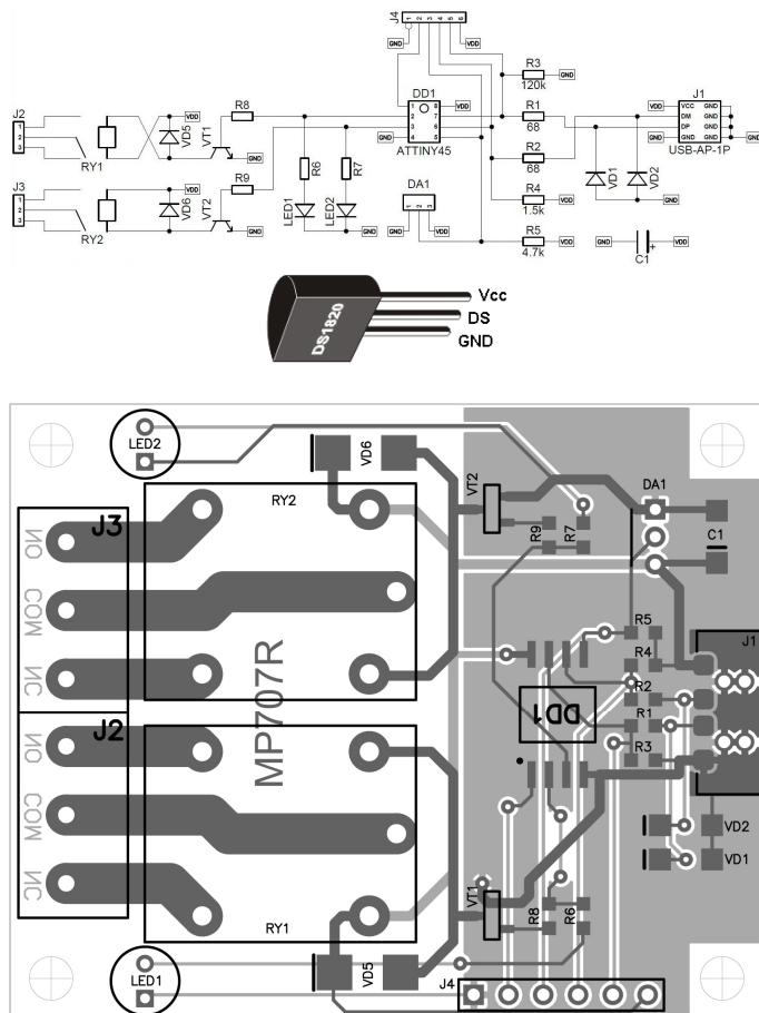
Рис..2 Схемы электрическая принципиальная и монтажная
