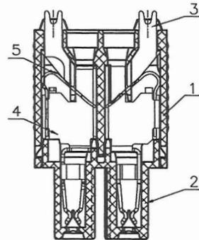
SEC A-A
