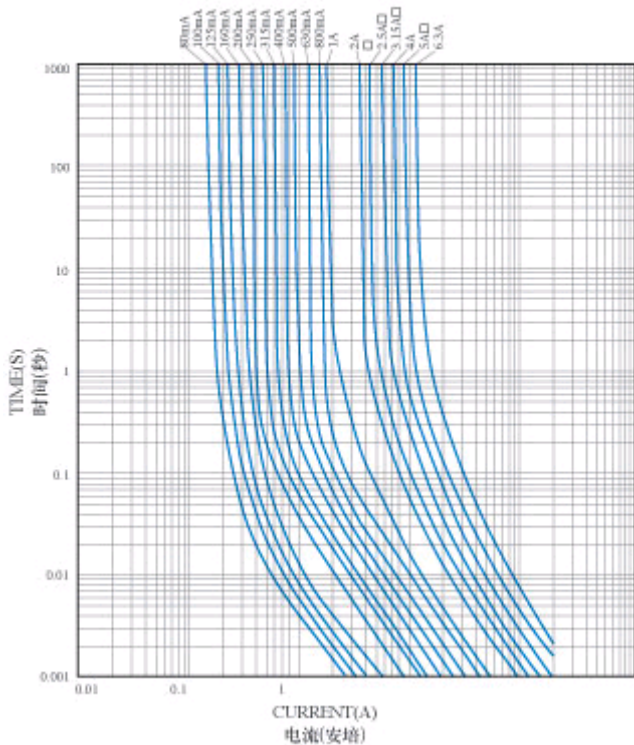
电流-时间曲线图
