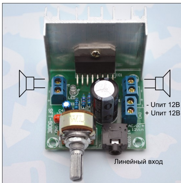
Рис.2 Назначение разъемов
