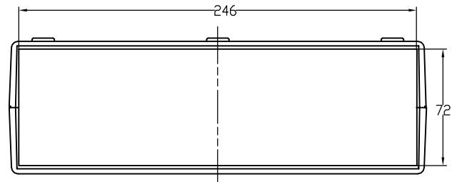
前面板尺寸
