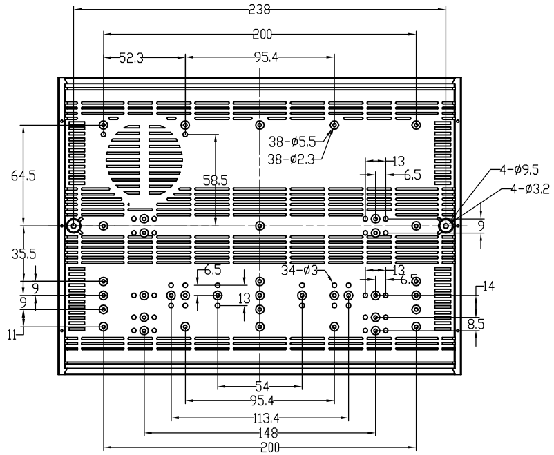
下盖正视图
