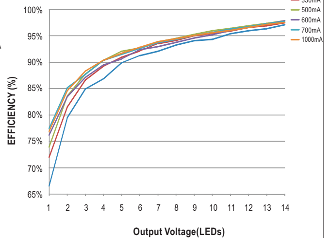
Fig-4 48VDC input, 1~14 LEDs(Vf=3V)
