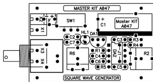
Рис.3 Монтажная схема
