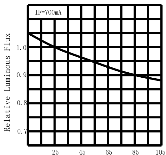
温度-相对光通量曲线
