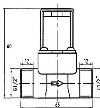
Установочные размеры
