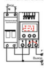
Монтажная схема
