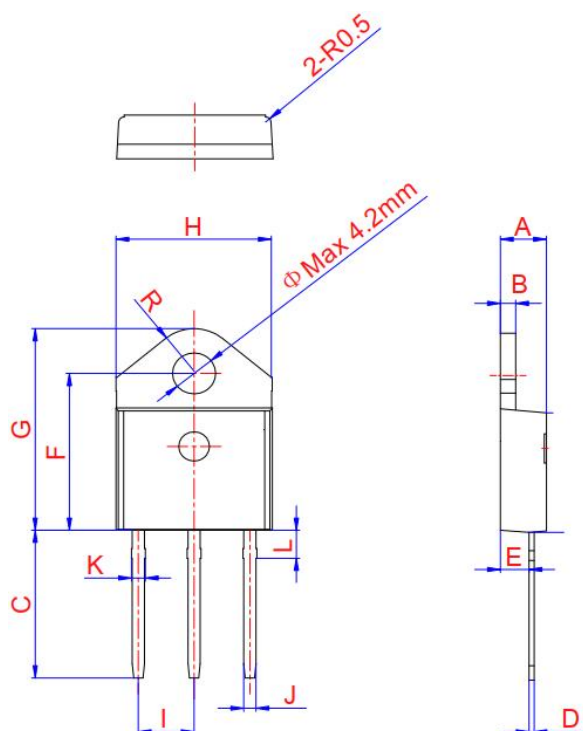
TO-3P Ins
