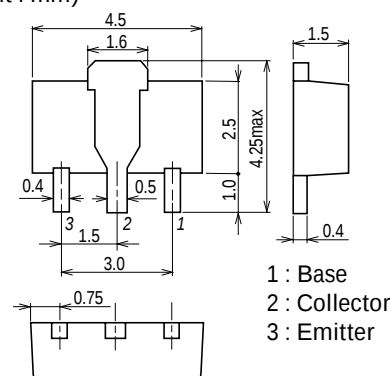
外形図 2038A
