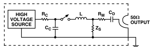
Figure 24. EFT Generator
