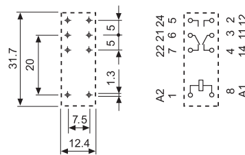
Вид сбоку
